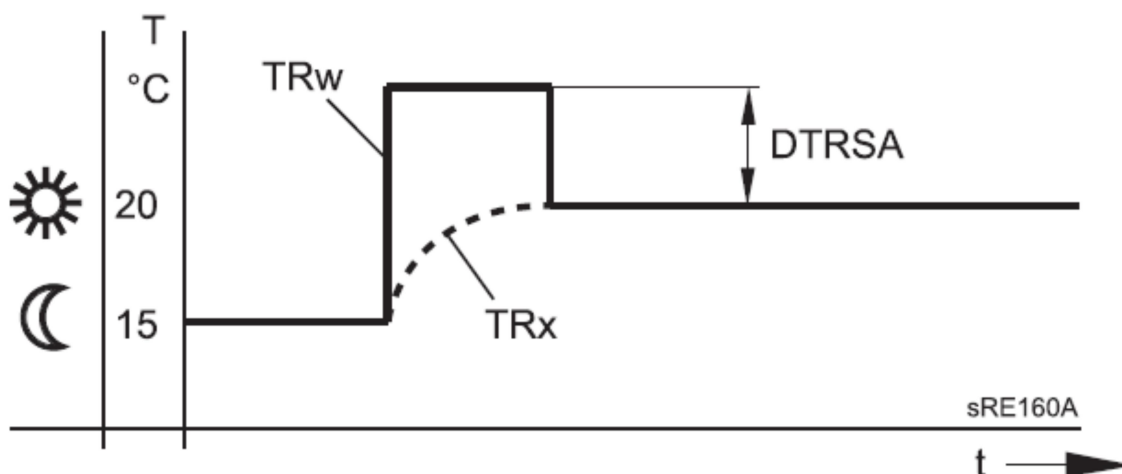
Рис.18 Ускоренное отопление
