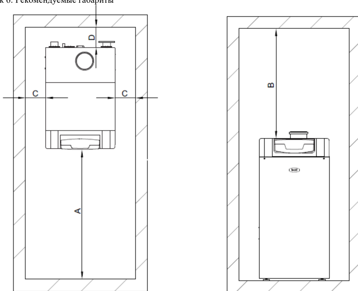
Рисунок 6: Рекомендуемые габариты
